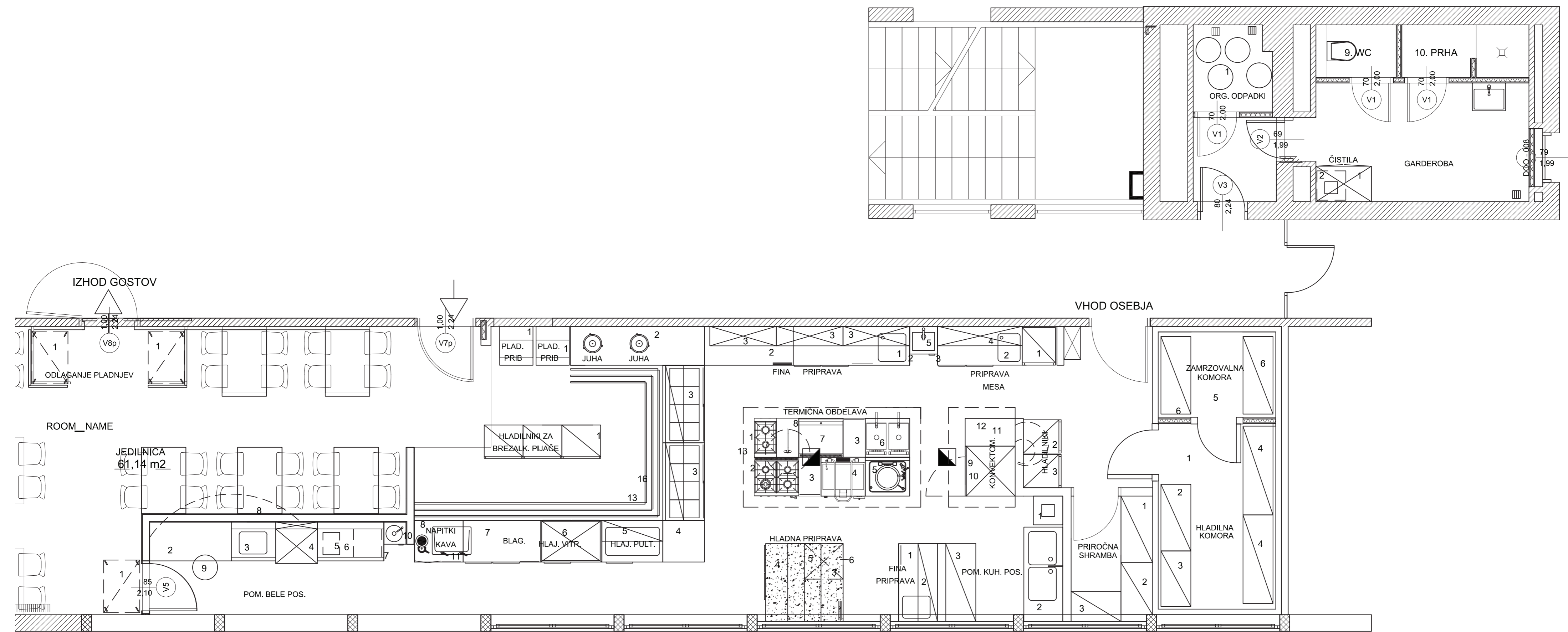
OBJEKT: FAKULTETA ZA STROJNIŠTVO V LJUBLJANI TEHNOLOŠKI RAZPORED KUHINJSKE OPREME
